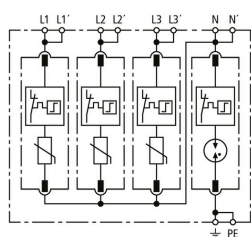
Schéma vnitřního zapojení DG MP TT 275 FM
