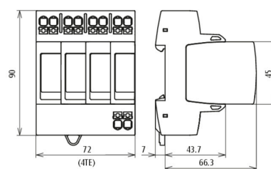
Rozměry DG MP TT 275 FM
